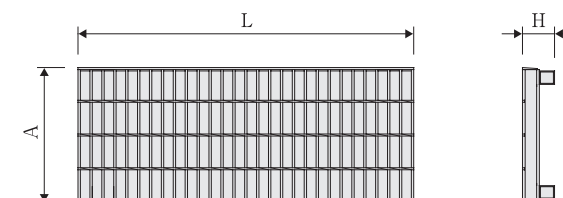
■グレーチング蓋
