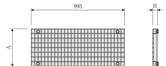
■グレーチング蓋 (T-25)
