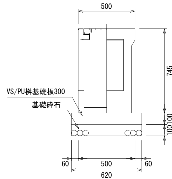
自由勾配側溝用桷 300×300×300
