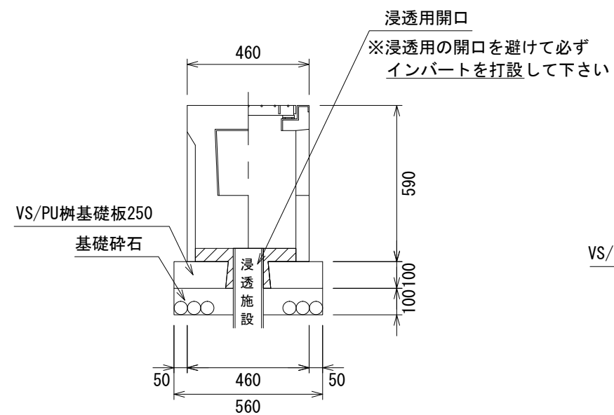
道路側溝用桷250
