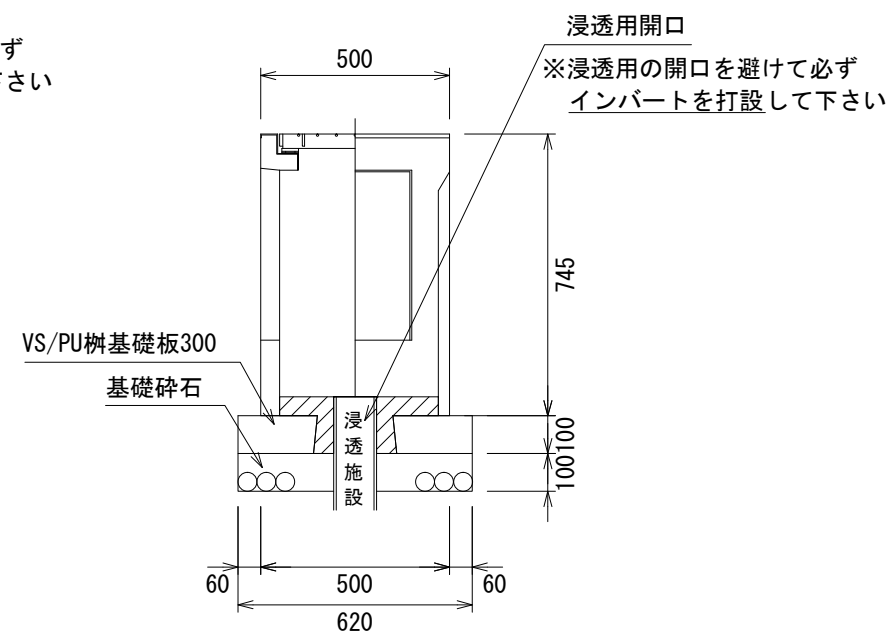
自由勾配側溝用桷 300×300×300
