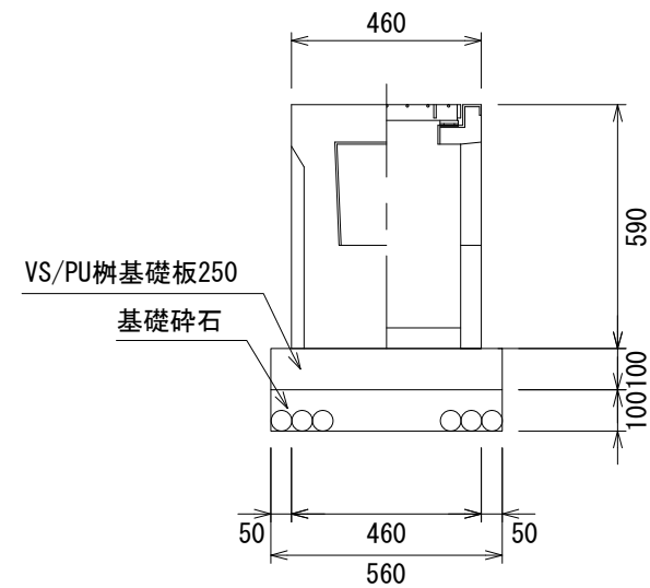
道路側溝用桷250
