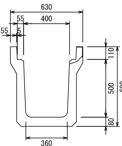
オメガ側溝3種400B
