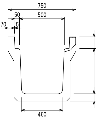
オメガ側溝3種500A
