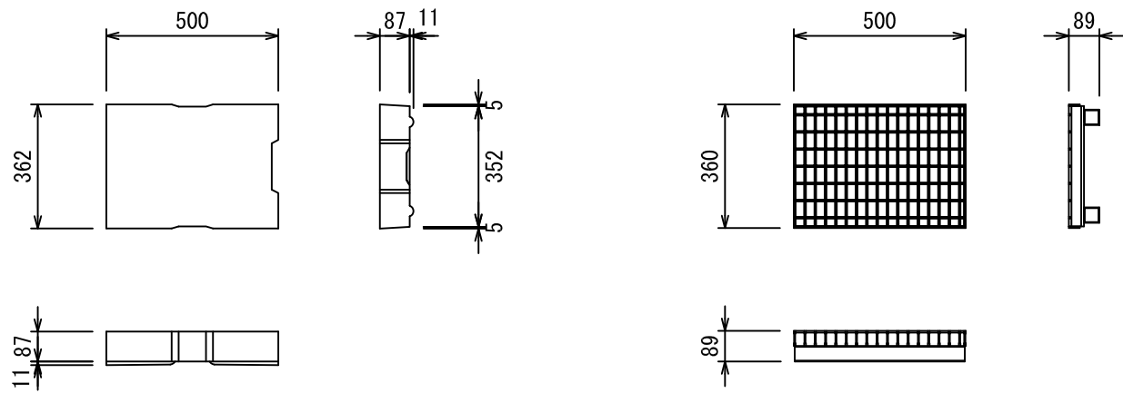
コンクリート蓋 3種250
