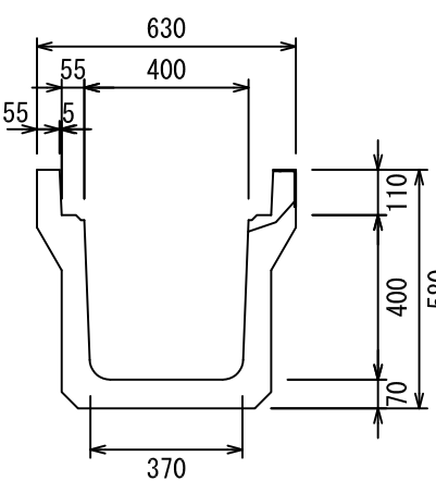
オメガ側溝3種400A
