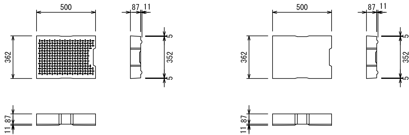
コンクリート蓋 3種250(スタッド20)
