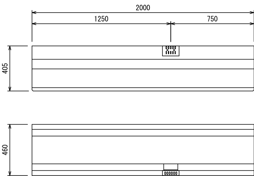
オメガ側溝3種製品図 S=1/20
