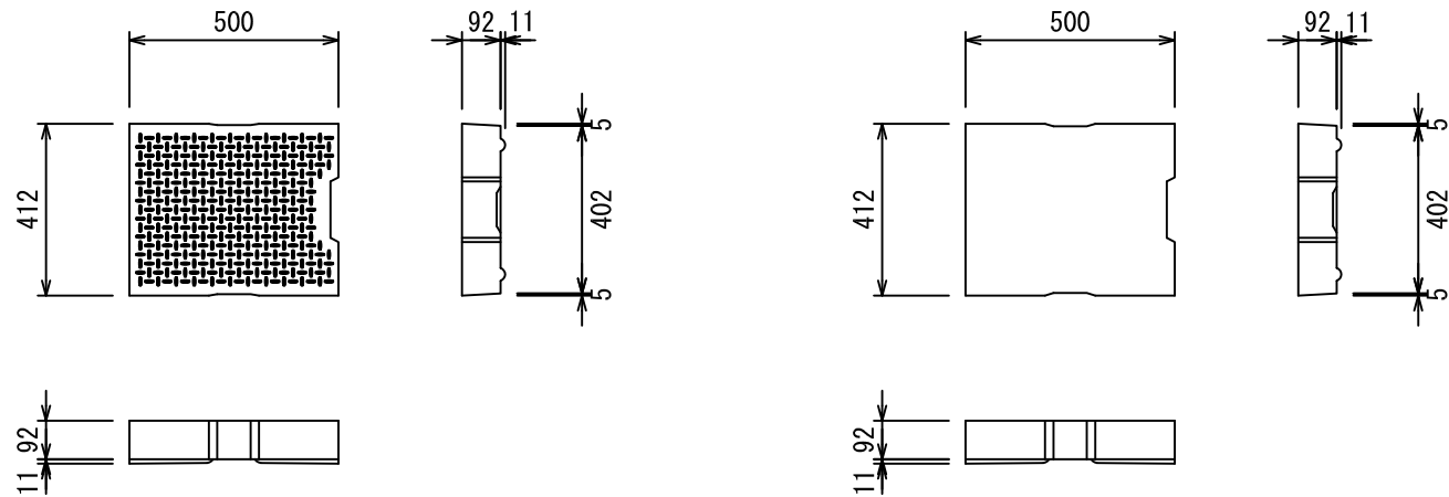
コンクリート蓋 3種300(スタッド20)
