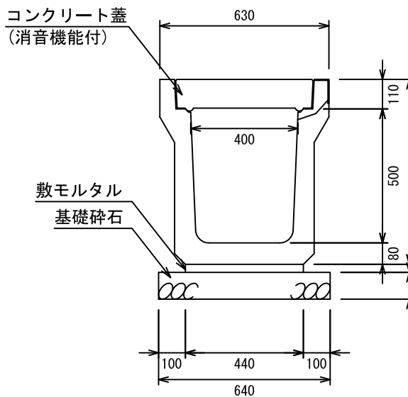
オメガ側溝 3種400B
