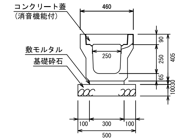
オメガ側溝 3種250
