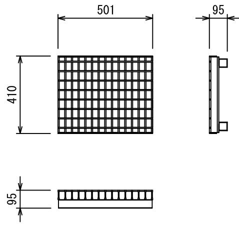
グレーチング蓋 300用(T-25)
