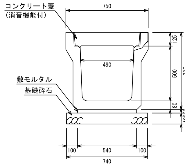
オメガ側溝 3種500A
