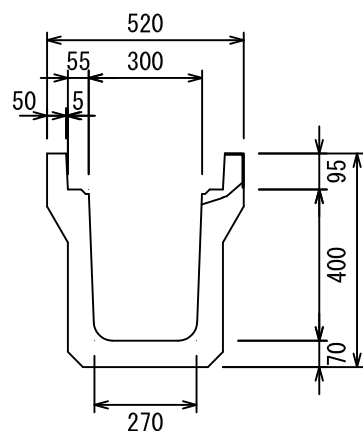
オメガ側溝3種300B
