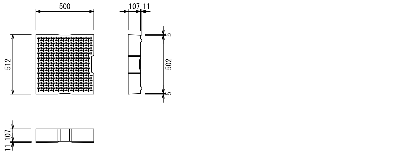
コンクリート蓋 3種400(スタッド20)
