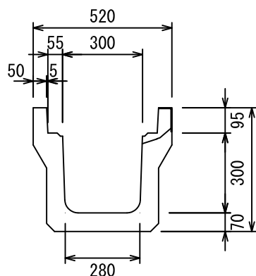
オメガ側溝3種300A
