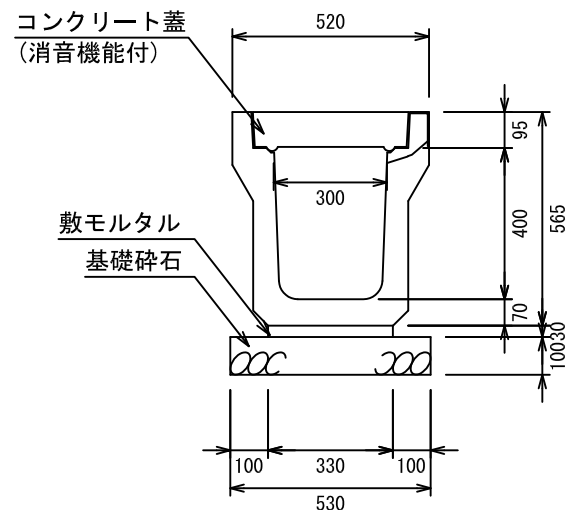
オメガ側溝 3種300B
