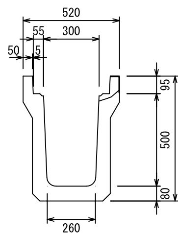
オメガ側溝3種300C
