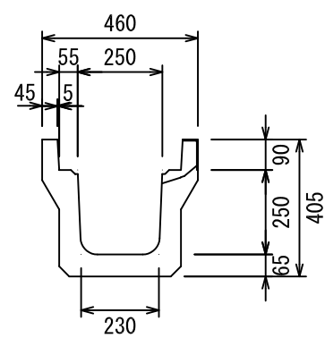
オメガ側溝3種250
