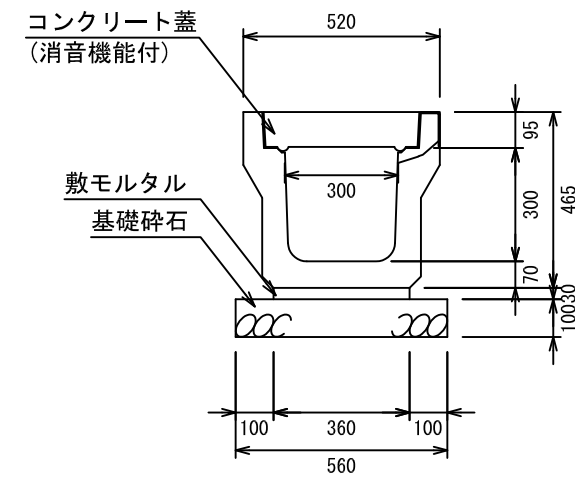
オメガ側溝 3種300A
