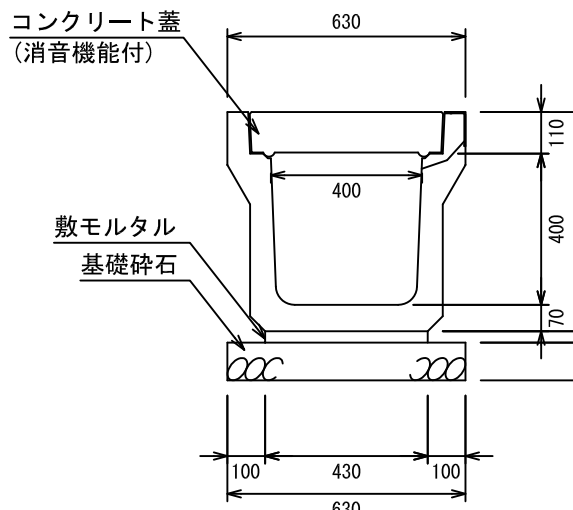
オメガ側溝 3種400A
