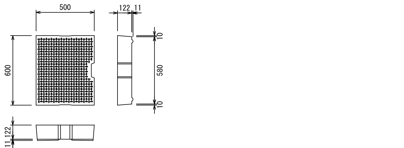
コンクリート蓋 3種500(スタッド20)
