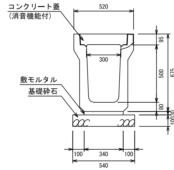
オメガ側溝 3種300C
