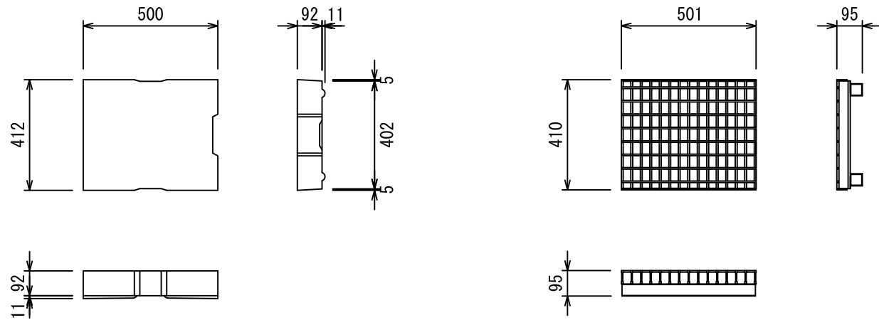
コンクリート蓋 3種300
