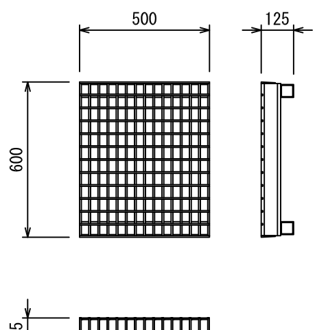
グレーチング蓋 500用(T-25)
