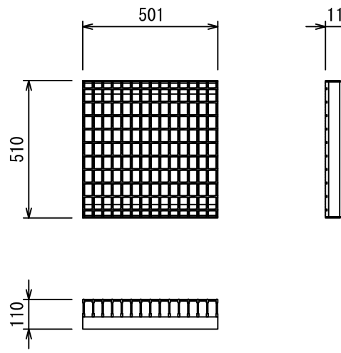
グレーチング蓋 400用(T-25)
