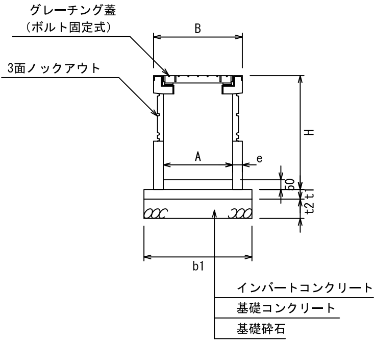
断面図
