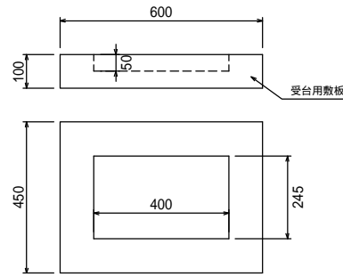
受台用敷板300
