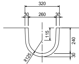
鉄筋コンクリートフリーム 250 L=3995
