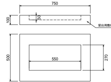
受台用敷板400
