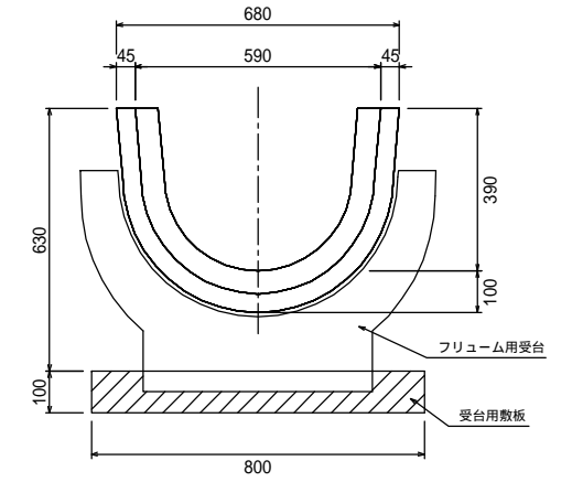
鉄筋コンクリートフリーム 450 L=3995
