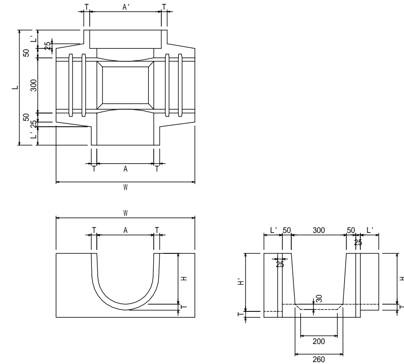
製品寸法表
