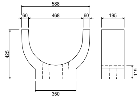
フリーム用受台300
