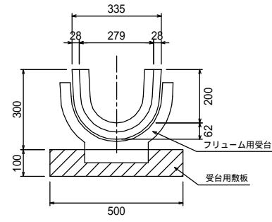
鉄筋コンクリートフリーム 200 L=3995
