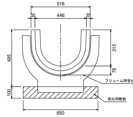
鉄筋コンクリートフリーム 350 L=3995
