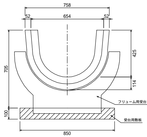
鉄筋コンクリートフリーム 500 L=3995
