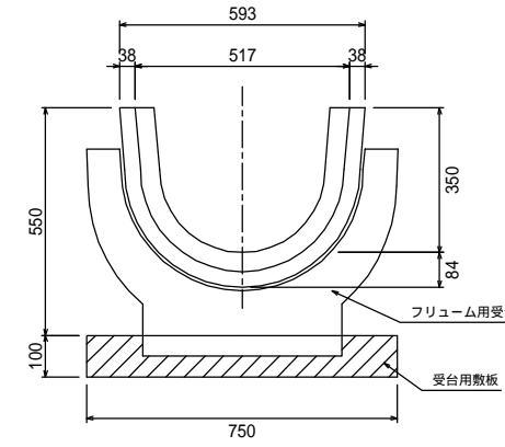
鉄筋コンクリートフリーム 400 L=3995
