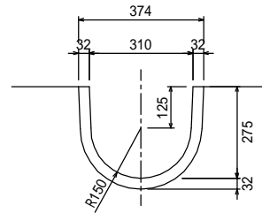
鉄筋コンクリートフリーム 300 L=3995
