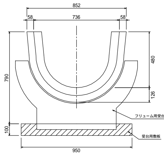
鉄筋コンクリートフリーム 560 L=3995
