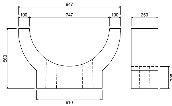
受台用敷板500
