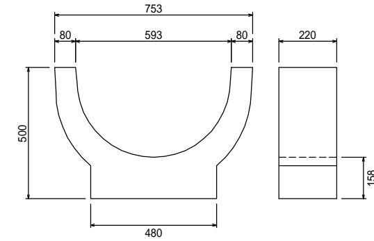
受台用敷板400
