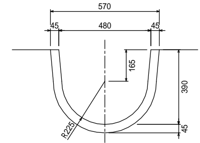
鉄筋コンクリートフリーム 450 L=3995
