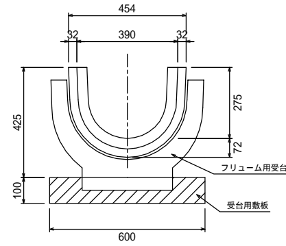
鉄筋コンクリートフリーム 300 L=3995
