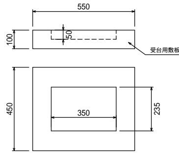
受台用敷板250
