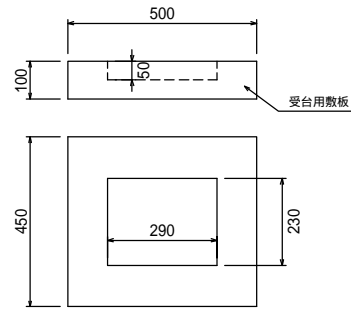
受台用敷板200
