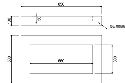
受台用敷板500
