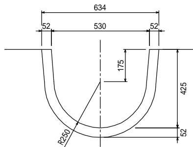
鉄筋コンクリートフリーム 500 L=3995
