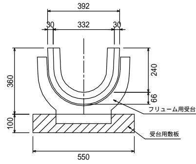
鉄筋コンクリートフリーム 250 L=3995
