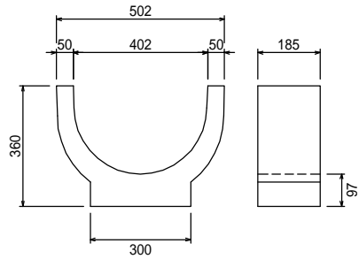
フリーム用受台250
