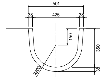
鉄筋コンクリートフリーム 400 L=3995
