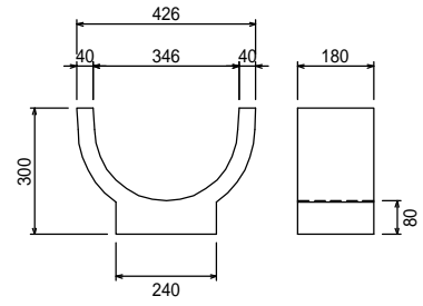
フリーム用受台200
