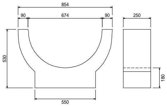
受台用敷板450
