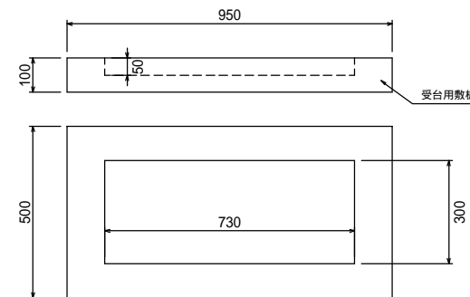
受台用敷板560
