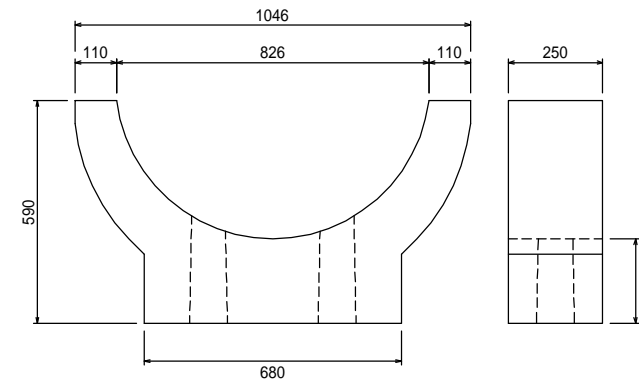
受台用敷板560
