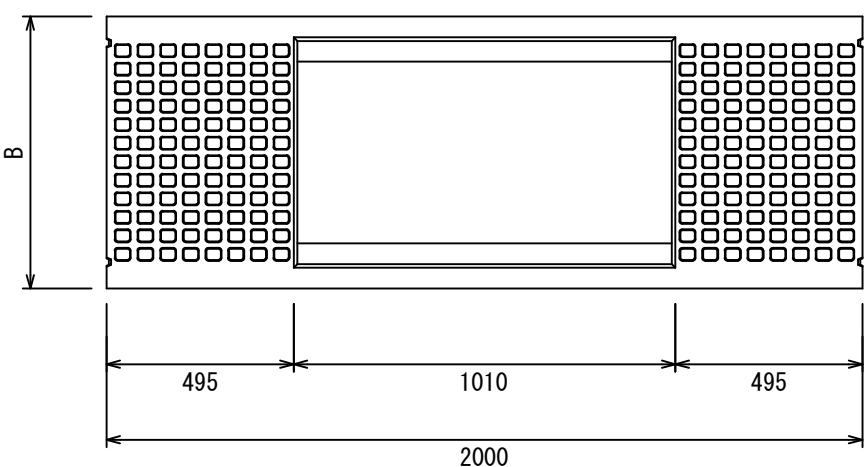
断面寸法
