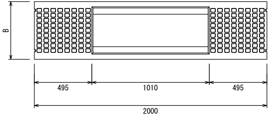
平面図
