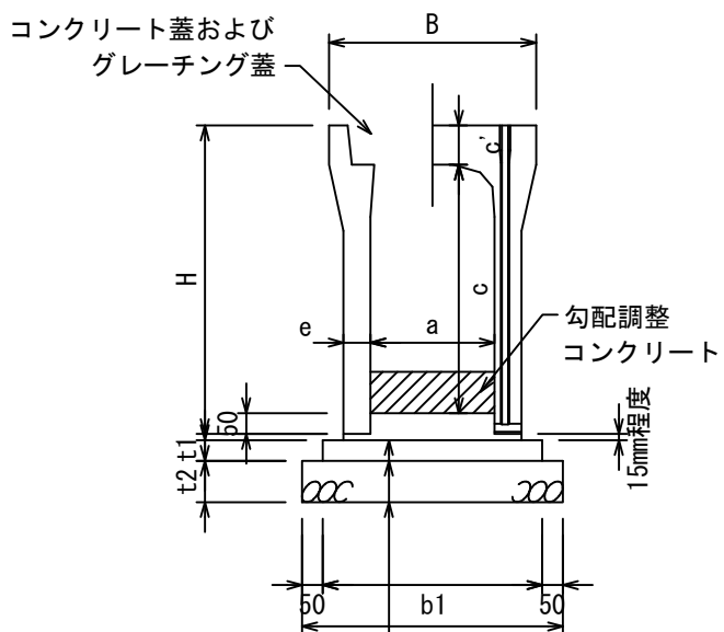
断面図
