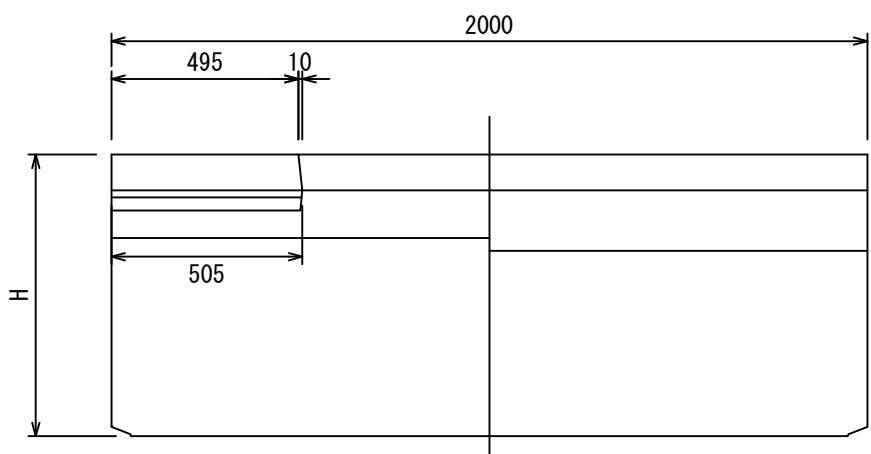
平面図
