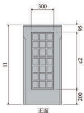
自由勾配側溝用柵(長方形) 製品寸法・重量表
