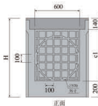
自由勾配側溝用柵(長方形) 製品寸法・重量表
