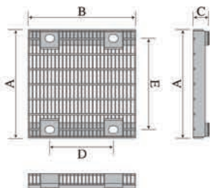
自由勾配側溝用枳グレーチング 寸法・重量表 (細目-T-25) 単位(mm)
