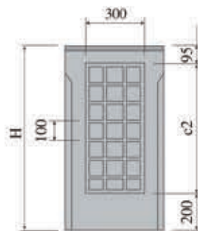
自由勾配側溝用柵(長方形) 製品寸法・重量表
