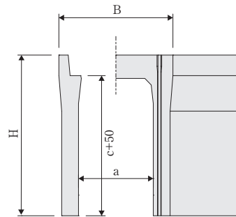
■側溝本体 (縦断面)
