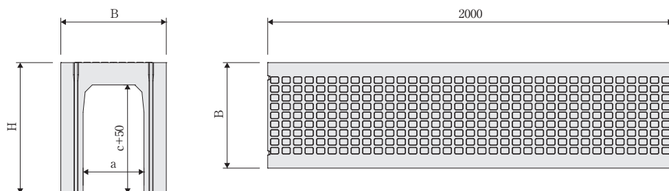
■側溝本体
