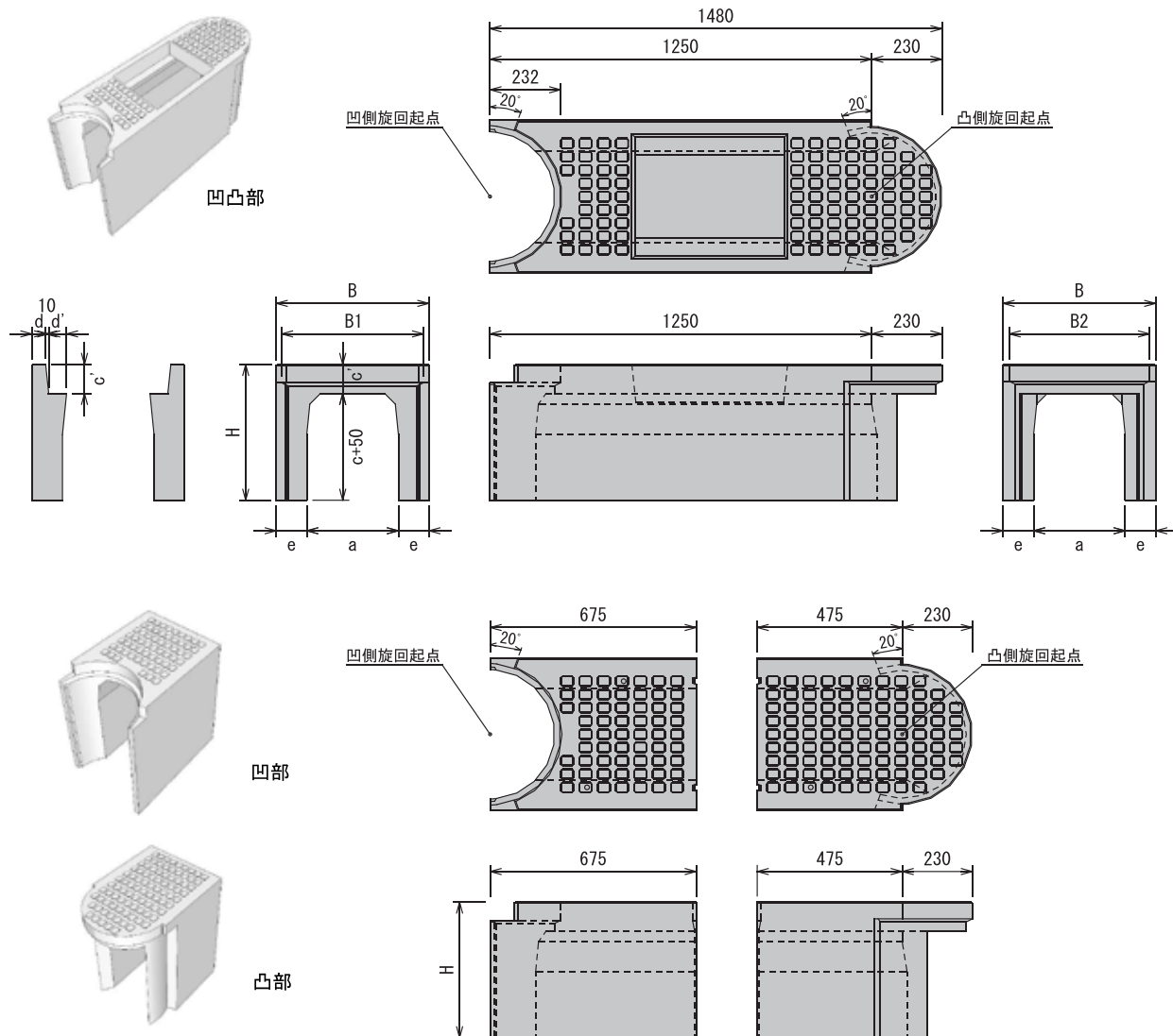
■寸法重量表
