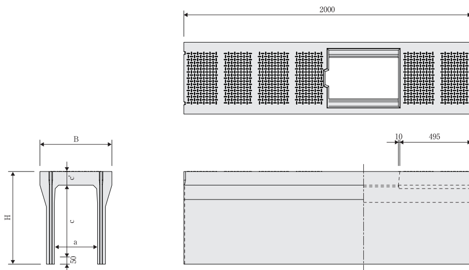
■寸法重量表
