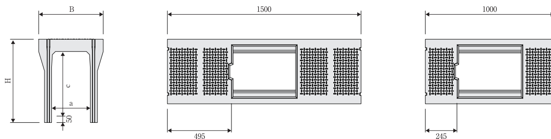
■寸法重量表 ※長さ1.5m製品
