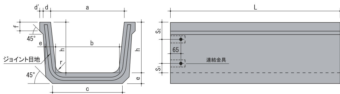
■寸法重量表
