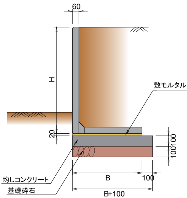
施工図
